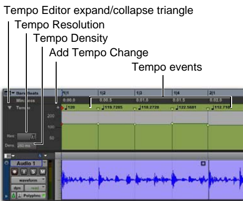
Tempo Editor
